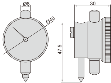
Reloj comparador
