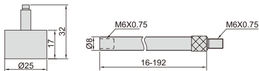
Bloque de equilibrio
